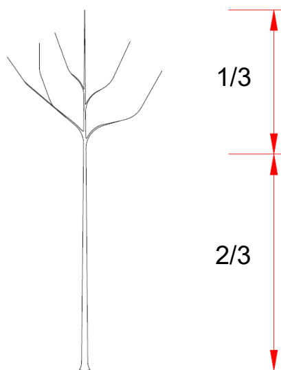
Obr. 3 Maximální poměr délky kmene a koruny při naplňování požadavku definovaného volného profilu koruny (5.1.3.9 a 5.2.3.1).
