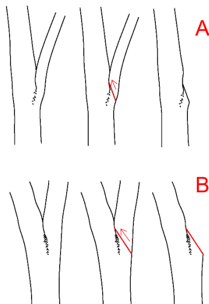
Obr. 4 Řez „tlakového“ větvení (4.1.11): A) schéma řezu boční větve v ostrém úhlu nasazení se zarůstající kůrou, B) řez kodominantního „V“ větvení (vidličnaté) se zarůstající kůrou.
