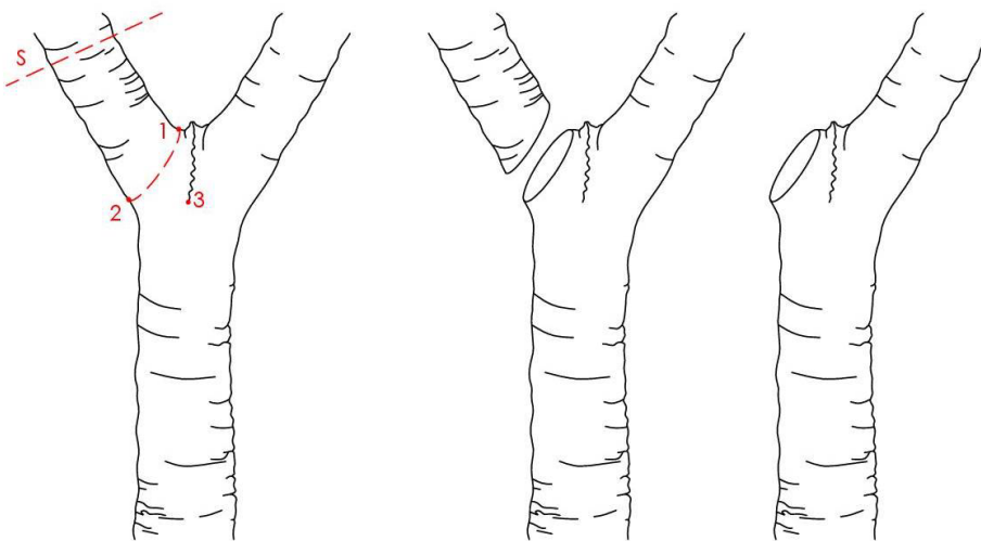
Obr. 7 Řez kodominantního „U“ větvení (tahové) s patrným korním hřebínkem (4.1.10): S - zakrácení odstraňované silné větve řezem „na tříkrát“, 1 – výchozí místo řezu těsně pod vrcholem korního hřebínku, 2 – koncový bod sklonu řezu v úrovni začátku tvorby korního hřebínku (bod 3)
